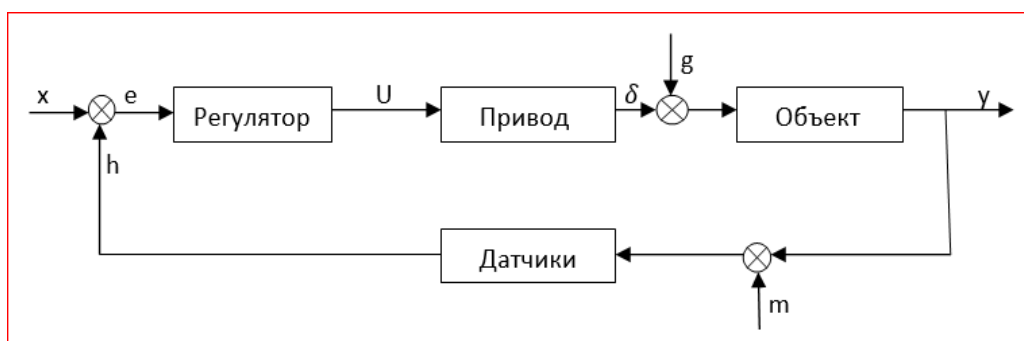
Фиг.1.1.Типовая схема управления с обратной связью. X- входной сигнал, e – параметр рассогласования, U-Сигнал управления, \delta - управляющее воздействие, g – помехи, искажающие управляющий сигнал, y – выходной параметр системы, m – помехи измерения выходного сигнала, h – сигнал обратной связи.
